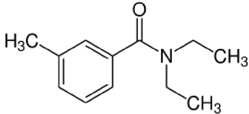
N,N - Dimetil–metatoluamida
