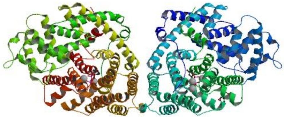
Limoneno Sintase
