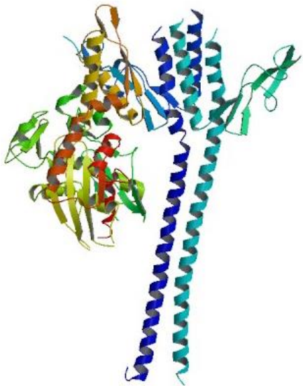
DnaK
