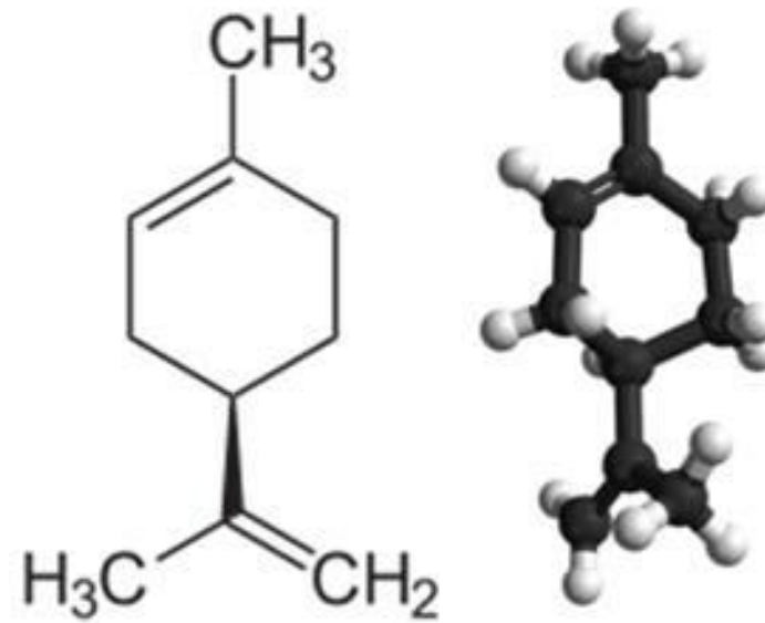
D-Limoneno
