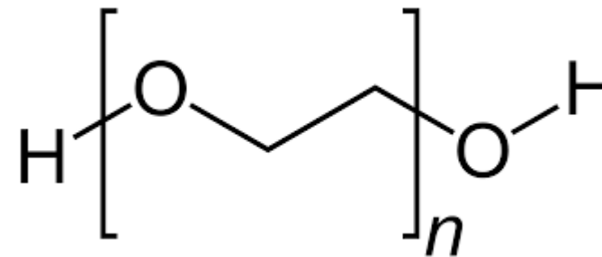
Polietilenoglicol (PEG)
